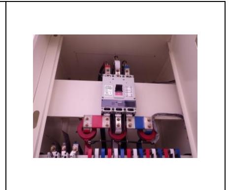
圖 4-3-3：主開關
