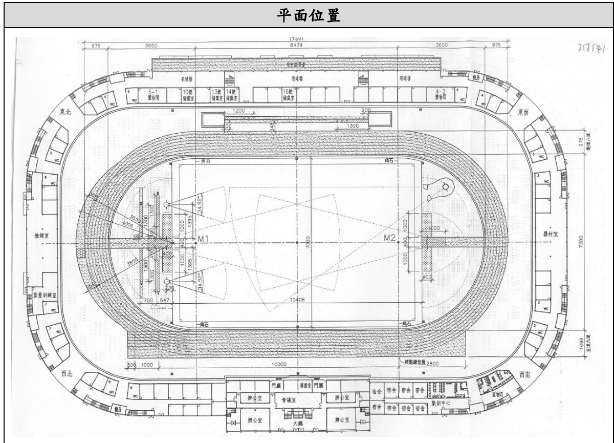
圖 1-2-1 彰化縣立田徑場場地平面圖
