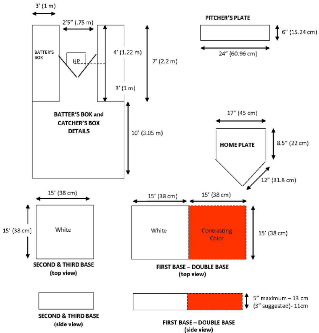
圖 5-5 投手板、本壘板、壘包和擊球區規格圖
