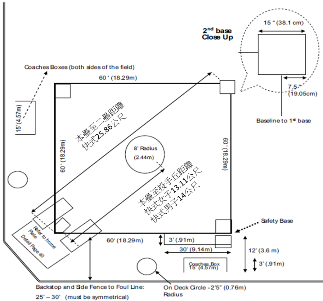
圖 5-3 正式壘球場方塊區之規格圖
