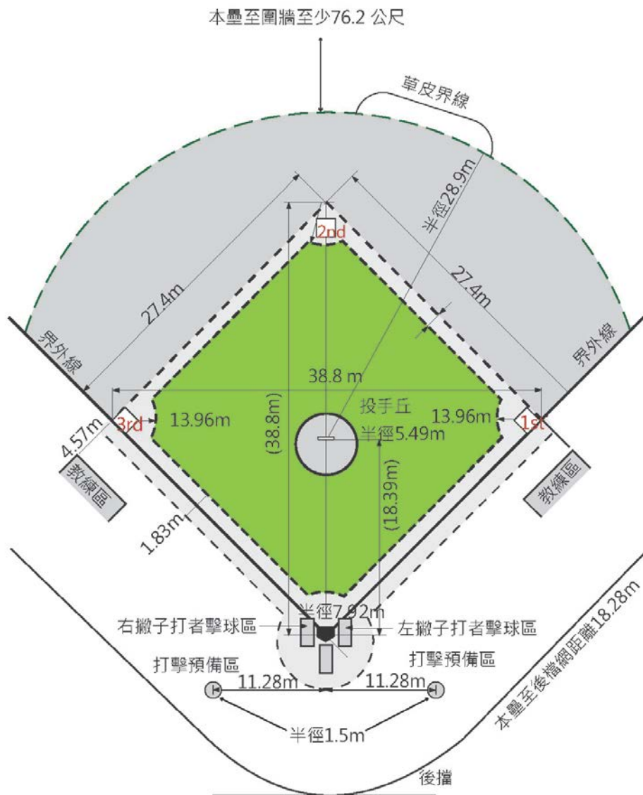
圖 5-1 棒球場內野布置圖
