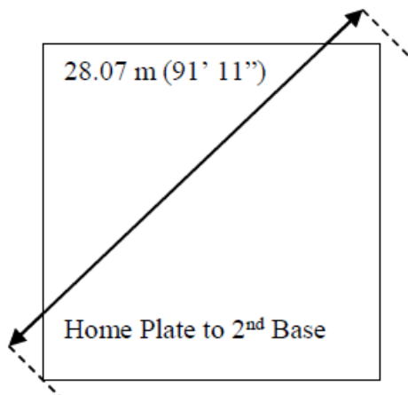
圖 5-4 慢式壘球 65 呎方塊區之簡圖
