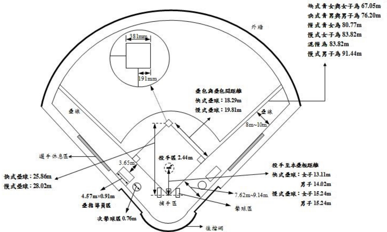
圖 5-2 正式壘球場之規格圖
