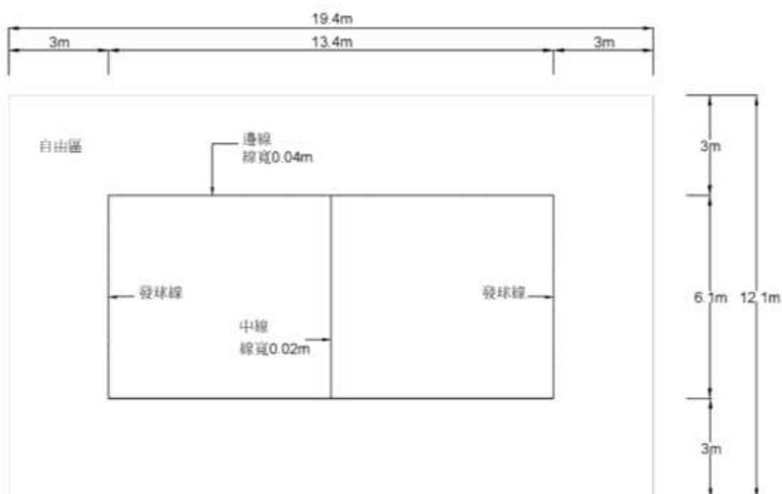
圖 26-1 藤球比賽場地尺寸
