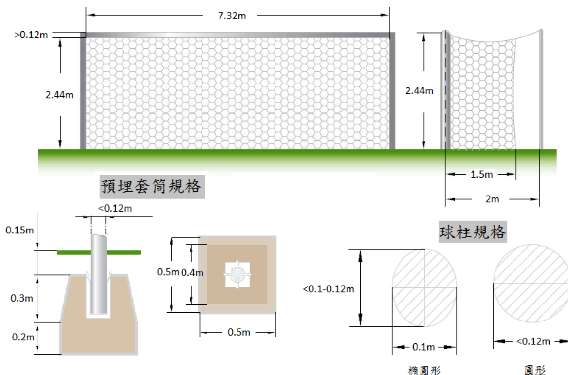
圖 14-2 足球門、球網、球柱設計圖
