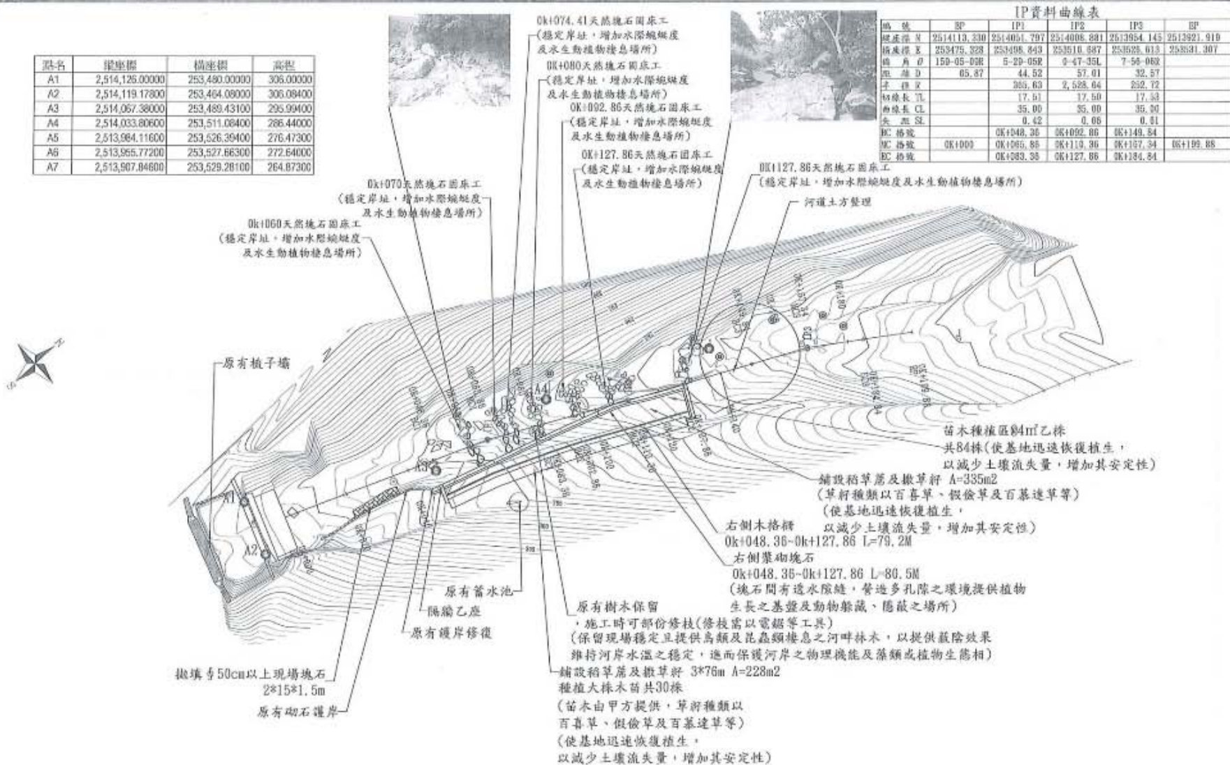
平面圖 S=1/1000
