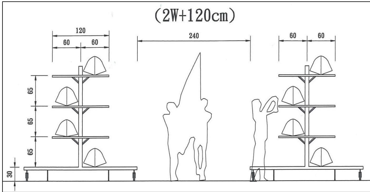
圖6-5 划船艇架雙向動線尺寸參考圖（單位：公分）
