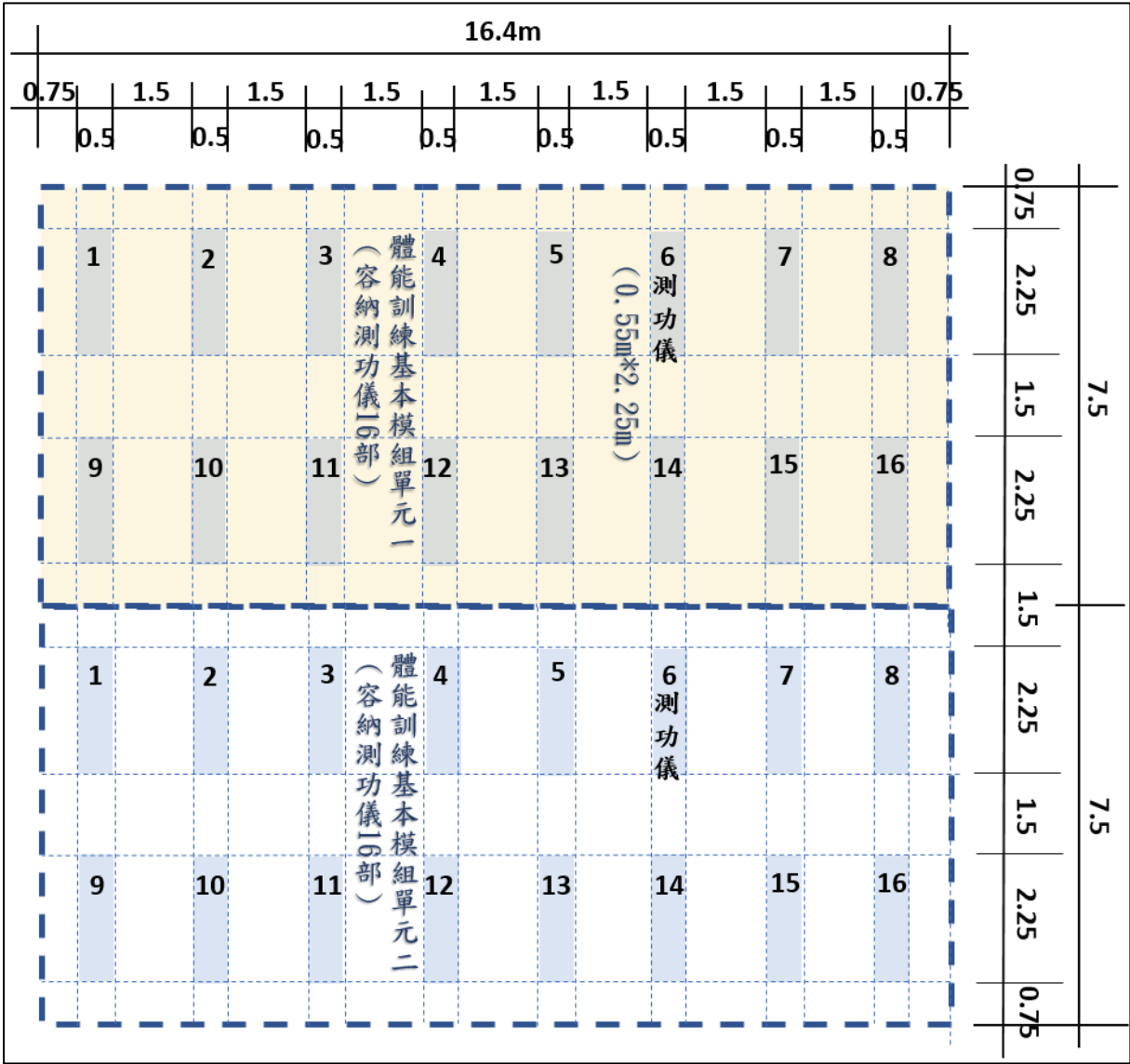
圖6-10 體能訓練空間基本模組單元
