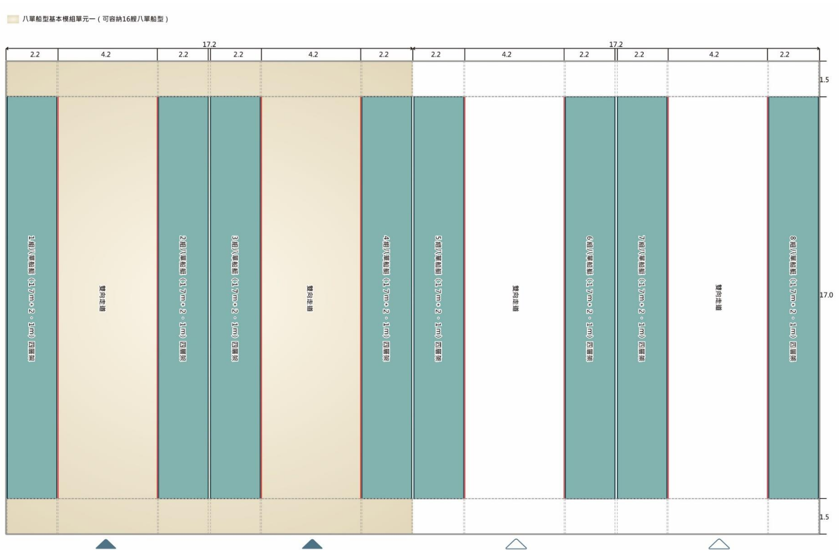
圖6-2 划船 Type C 場域艇庫基本模組單元圖
