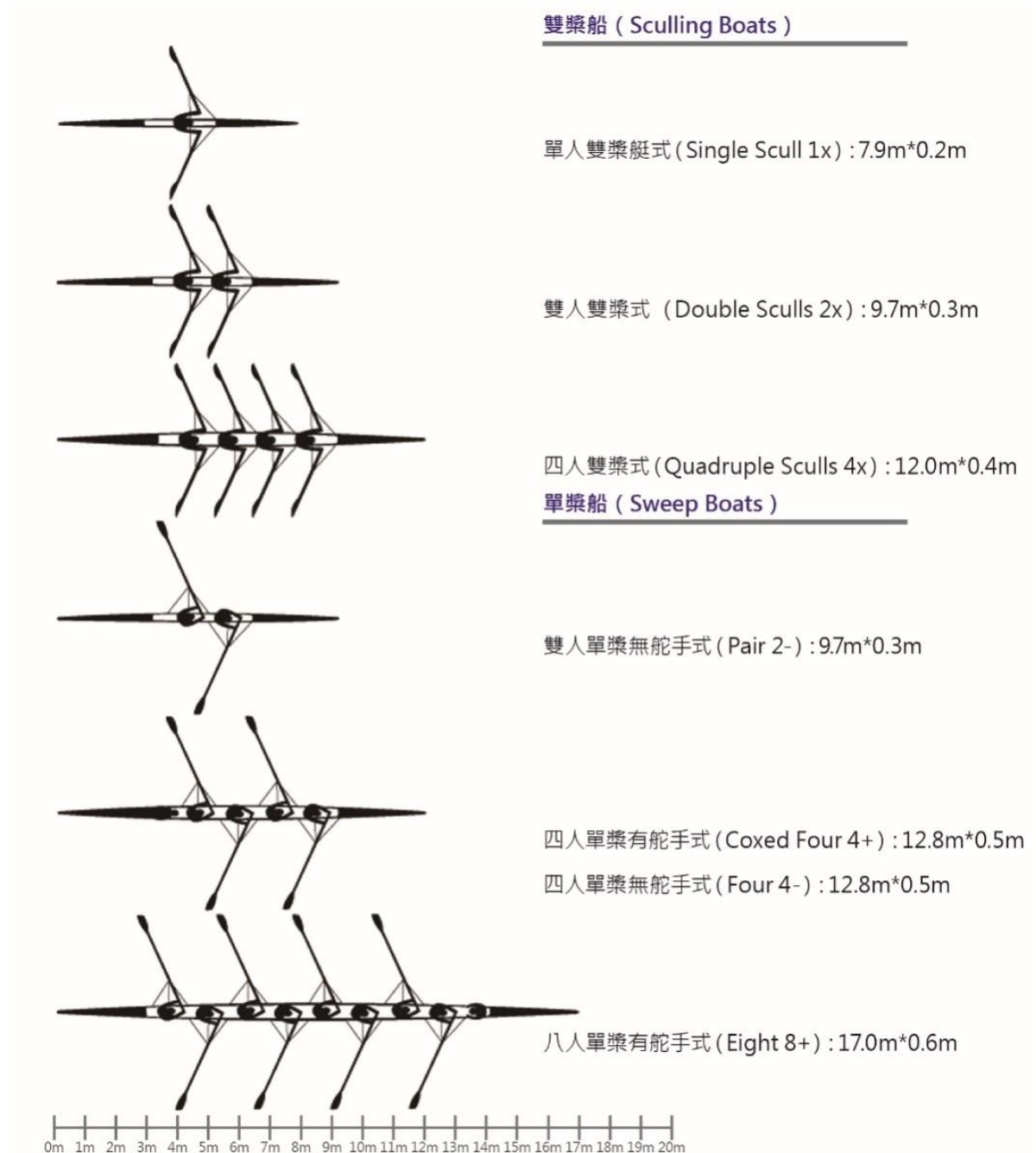
圖6-1 划船船型規格圖
