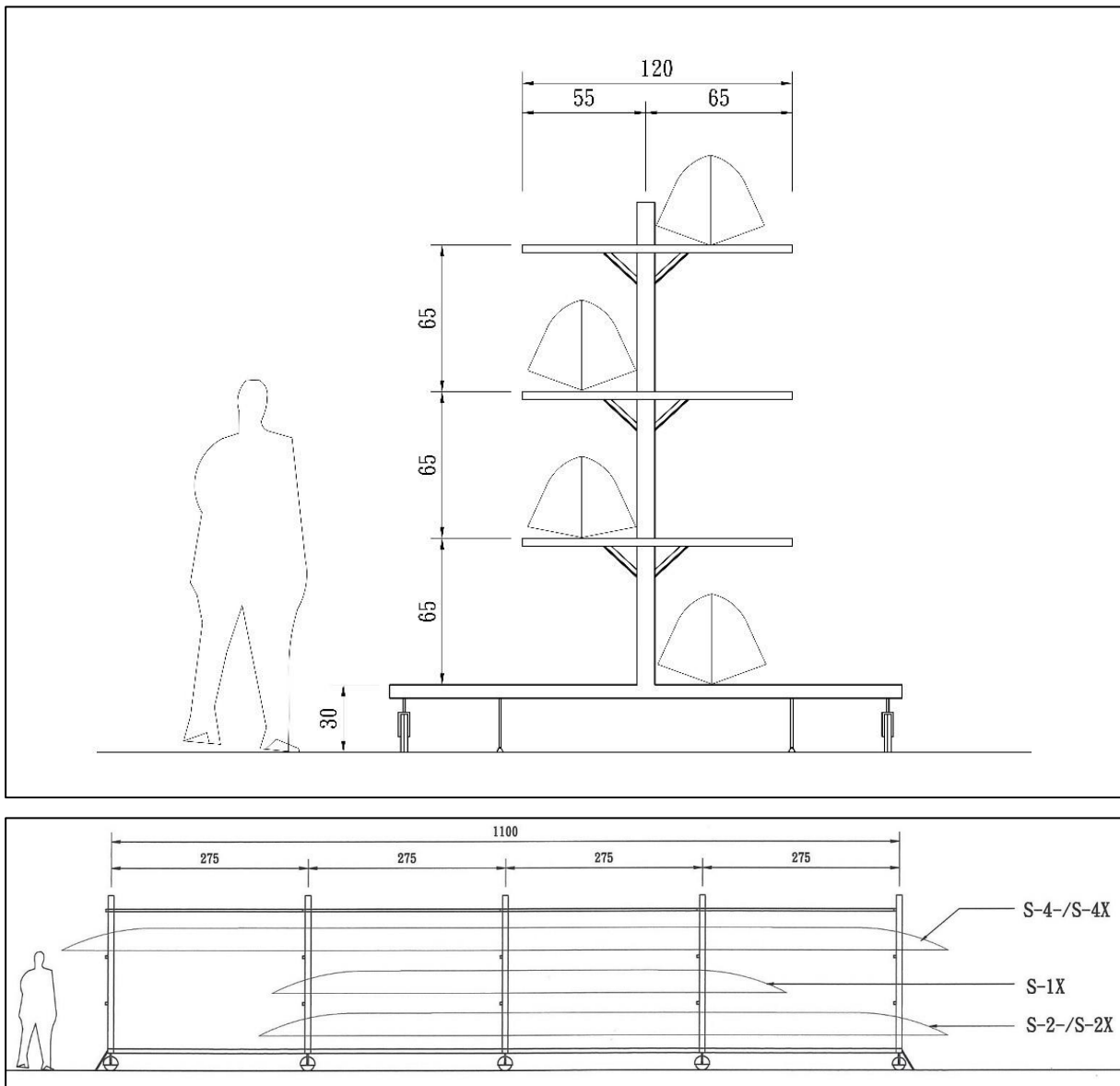
圖6-3 划船艇架示意圖（正立面-上圖、側立面-下圖；單位：公分）
