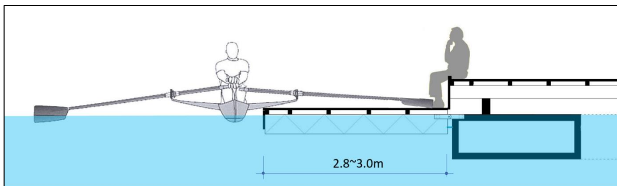
圖7-4 浮動平臺乾舷高與寬度示意圖
