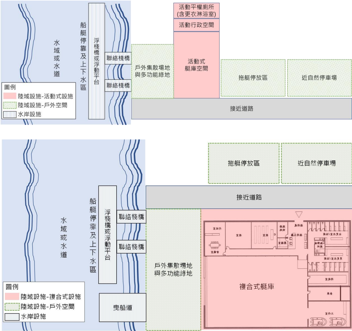
圖3-3 水域運動設施分類示意圖(活動式設施-上圖、複合式艇庫-下圖)
