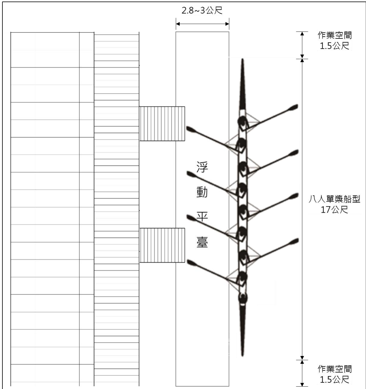
圖7-5 聯絡棧橋與浮動平臺連接平面示意圖
