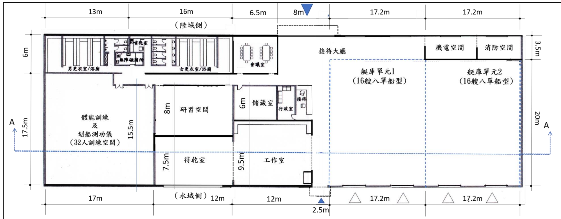
圖6-7 划船複合式艇庫平面配置示意圖
