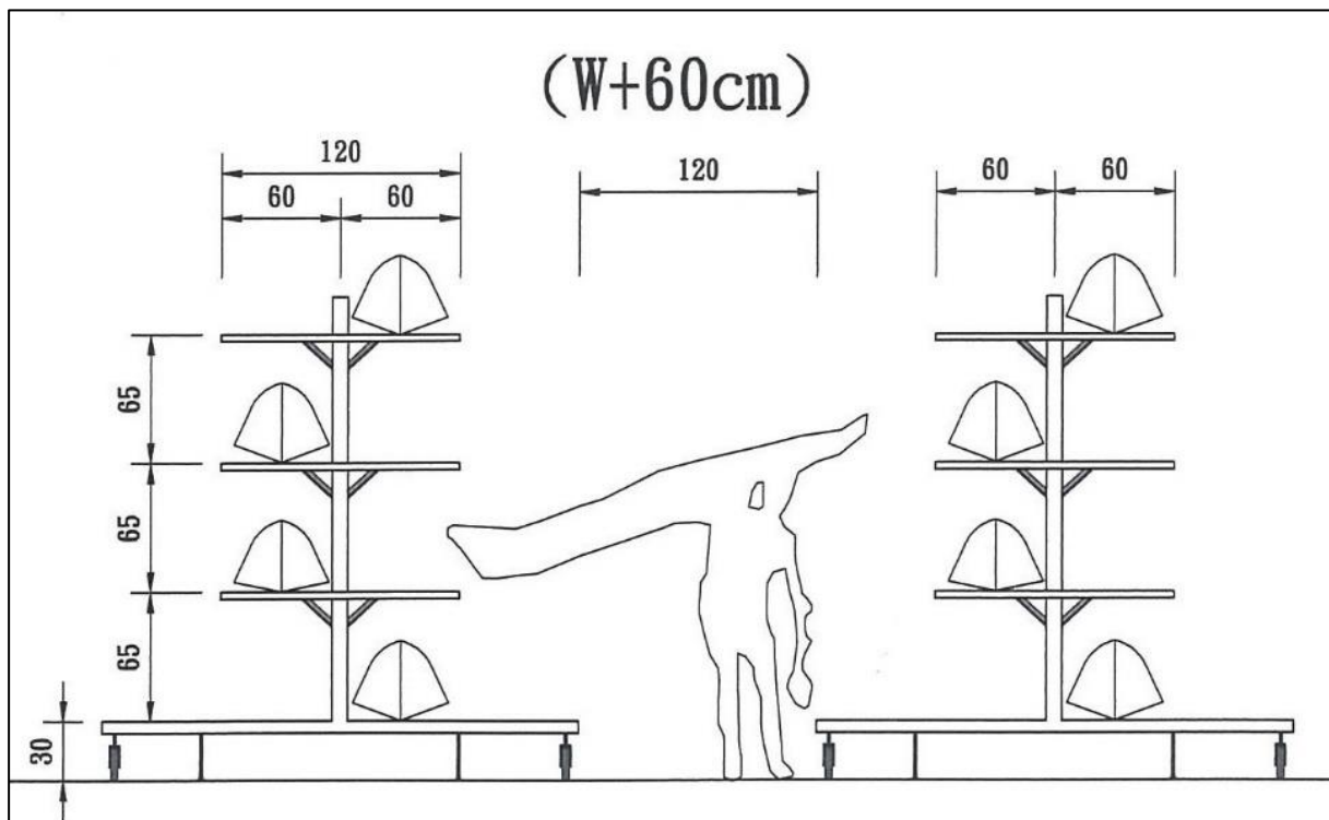
圖6-4 划船艇架單向動線尺寸參考圖 (單位：公分)
